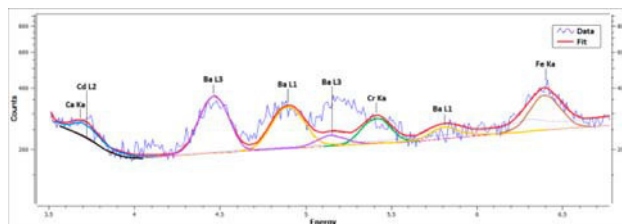
Figura 8. Determinación de elementos que componen los aditivos del PVC.
