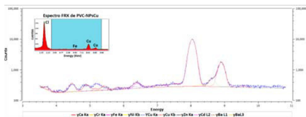
Figura 7. Espectro FRX de la muestra de PVC conteniendo NPsCu 0 .
