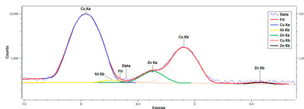
Figura 9. Determinación de Cobre en la muestra de PVC analizada
