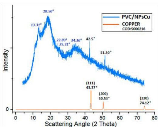
Figura 12. Patrón de difracción de la muestra obtenida de PVC/NPsCu 0 y patrón de difracción de Cu o .
