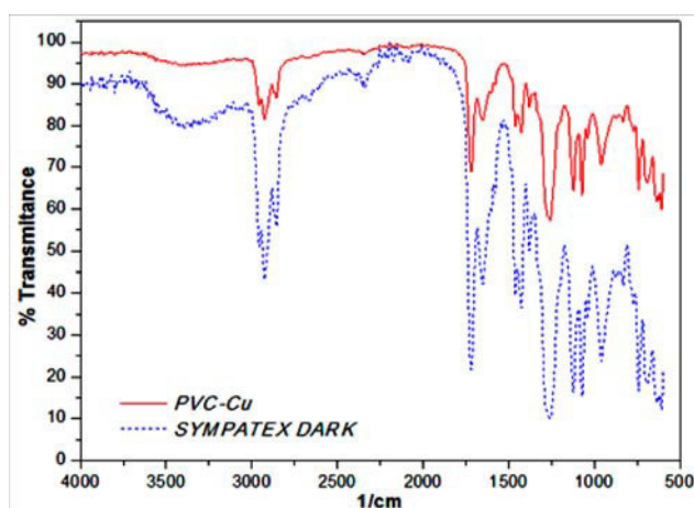
Figura 10. Espectro Infrarrojo por ATR del nanocompuesto PVC/NPsCu 0 , comparado con espectro SYMPATEX DARK de la base espectral NICODOM.IR.
