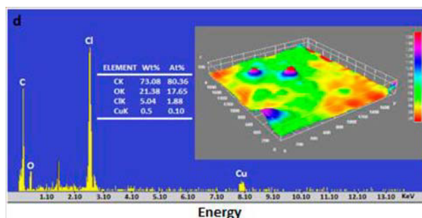
Figura 11. Caracterización de nanopartículas de cobre en la matriz polimérica de PVC: (a) 5 \mu\text{m} y (b) 2 \mu\text{m} de magnificación. (c) Muestra el histograma de distribución de tamaños de las nanopartículas por tratamiento de imagen. (d) Muestra el espectro EDS de nuestro nanocompuesto y una vista superficial del área estudiada.
