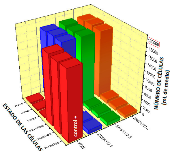
Figura 15. Representación gráfica del estudio citotóxico de los laminados de PVC/NPsCu en sangre periférica humana, concluyendo que el efecto citotóxico es menor al 8%.
