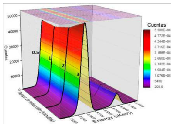
Figura 6. Análisis de la muestra de PVC/NPsCu 0 a diferentes tiempos de gelificación.
