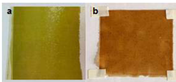
Figura 5. (a) Muestra previa a la gelificación de PVC. (b) Muestra gelificada de PVC por un tiempo de 2.5 minutos a 200°C, evidenciando la formación de NPS de Cu 0 .
