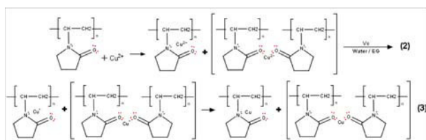
Figura 3. Ecuación de formación de complejo [\text{Cu}^{2+} - \text{PVP}] .
