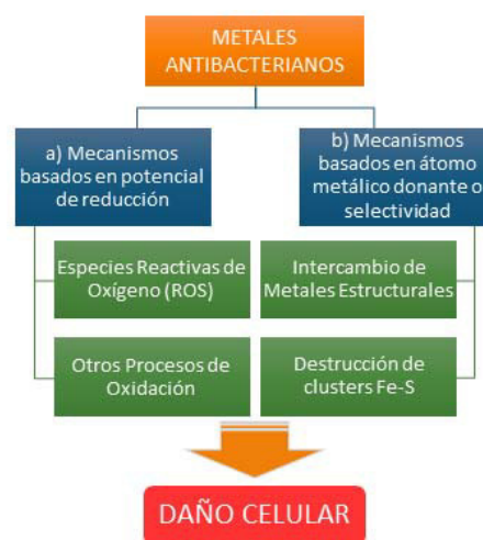
Esquema 1. Principales mecanismos que intervienen en la conducta antibacteriana de los metales de acuerdo a la propiedad del metal responsable de la acción: (a) El potencial de Reducción y (b) Selectividad del átomo donante.
