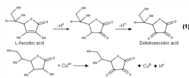
Figura 4. Ecuación y esquema de reacción de AA con \text{Cu}^{2+} .
