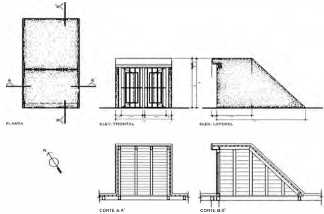
Gráf. 1. Dimensiones y características básicas de la teatina modelo.
