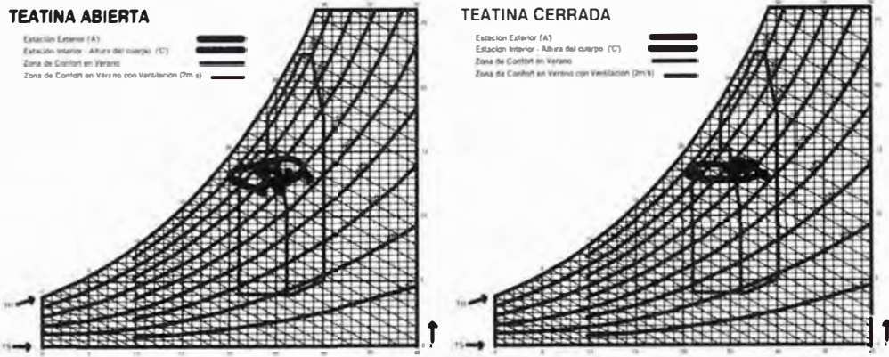
Gráf. 5. Datos de temperatura y humedad relativa del aire sobre el ábaco psicométrico considerando la abertura vertical de la teatina abierta (izquierda) y cerrada (derecha). Se representan las estaciones exterior (en azul) e interior (a nivel de la persona, en rojo). La prueba fue realizada durante días particularmente calurosos de la época de verano.
