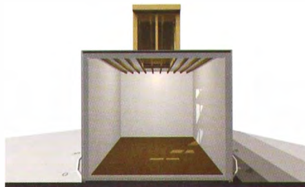
Gráf 3: Simulación en AutoCAD del mes de mayor ingreso de radiación solar directa a través de la teatina, diciembre.
