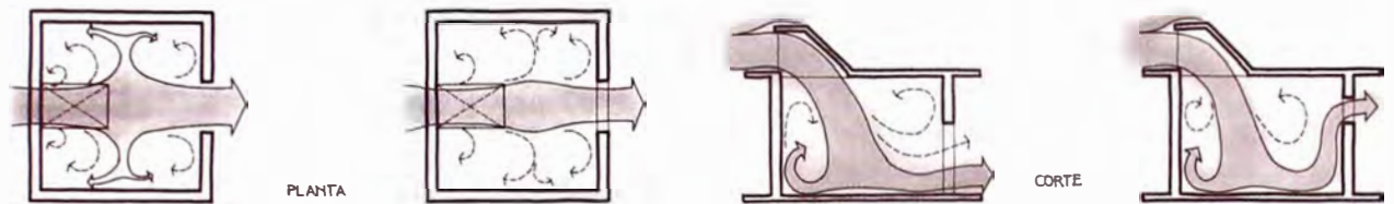
Gráf. 6: Patrón de recorrido típico del viento al interior de una habitación con teatina y puerta (izquierda) o ventana alta (derecha) frente a ella.
