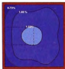
Gráf. 7. Distribución de la luz sobre el plano de trabajo de la habitación A.01.
