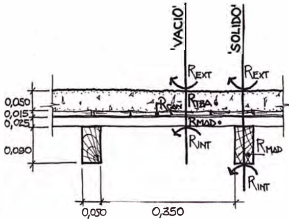
Gráf. 4: Esquema en corte de las diferentes resistencias térmicas del cerramiento de la teatina.
