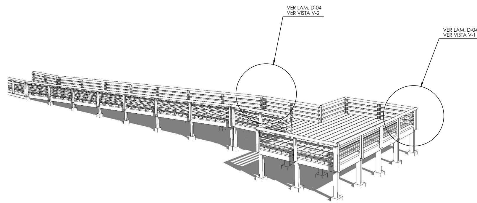
VISTA PERSPECTIVA ESTRUCTURA
