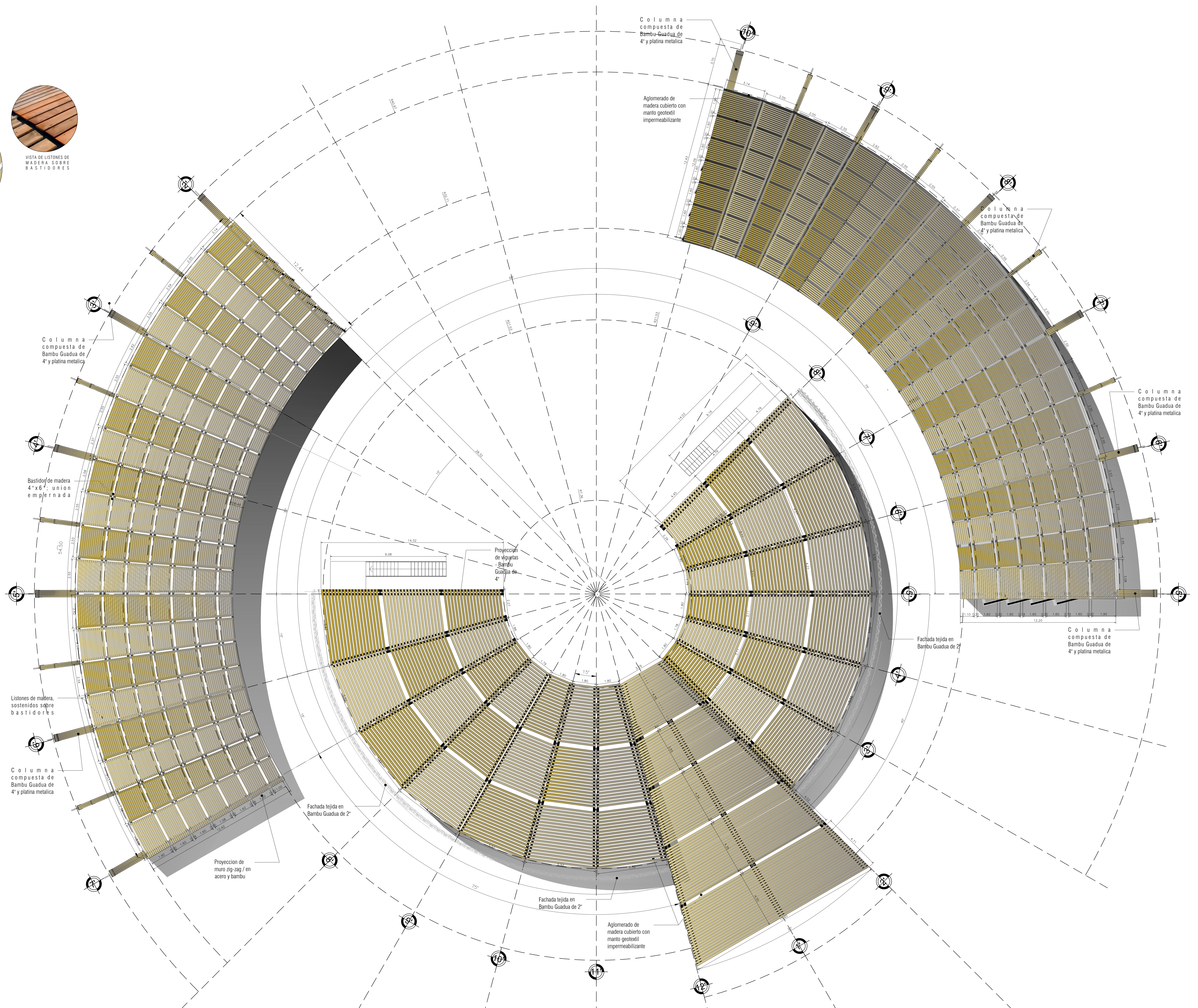
VISTA DE BASTIDORES UNIDOS MEDIANTE UNION METALICA
