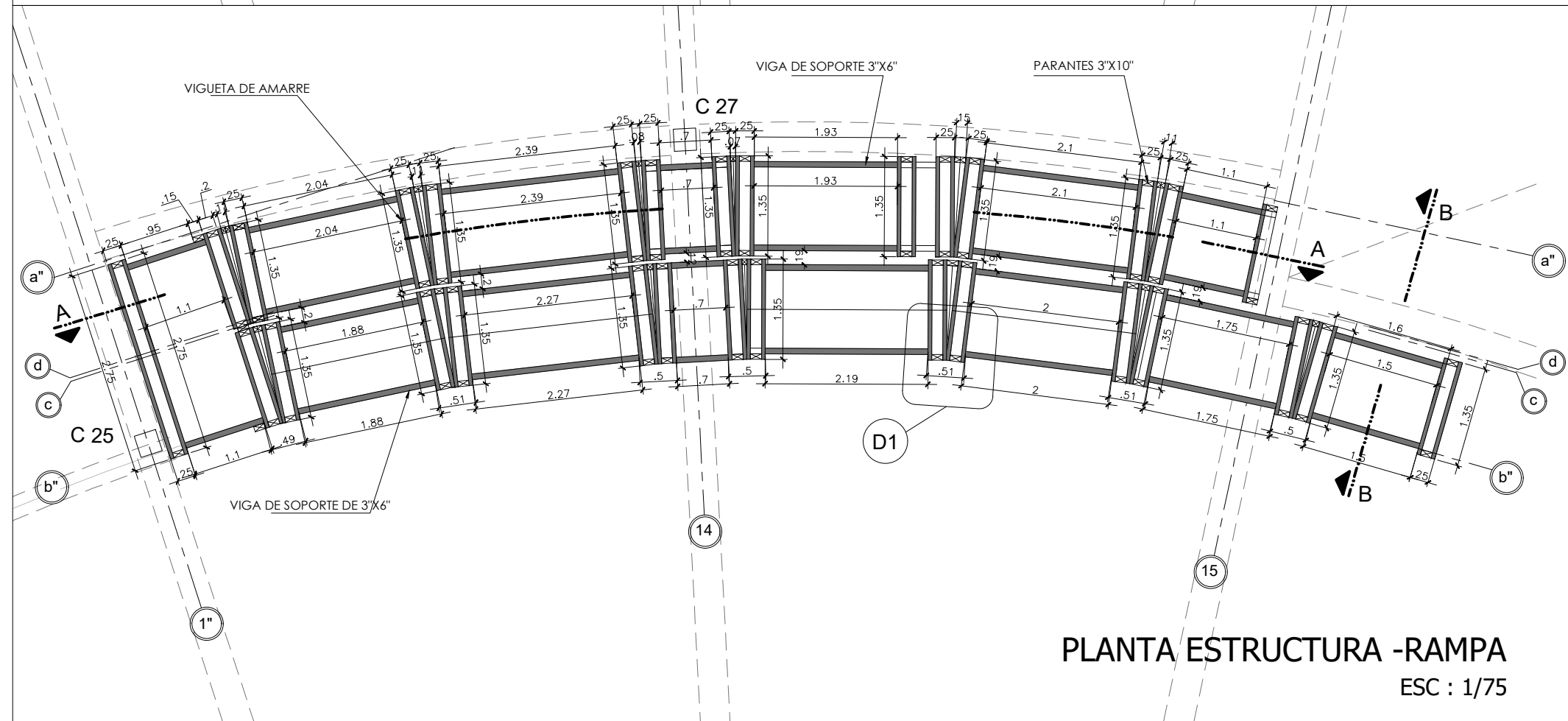
PLANTA RAMPA ESC : 1/75
