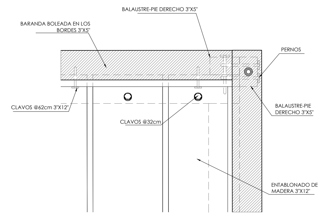
DETALLE E-1 ESC:1/10
