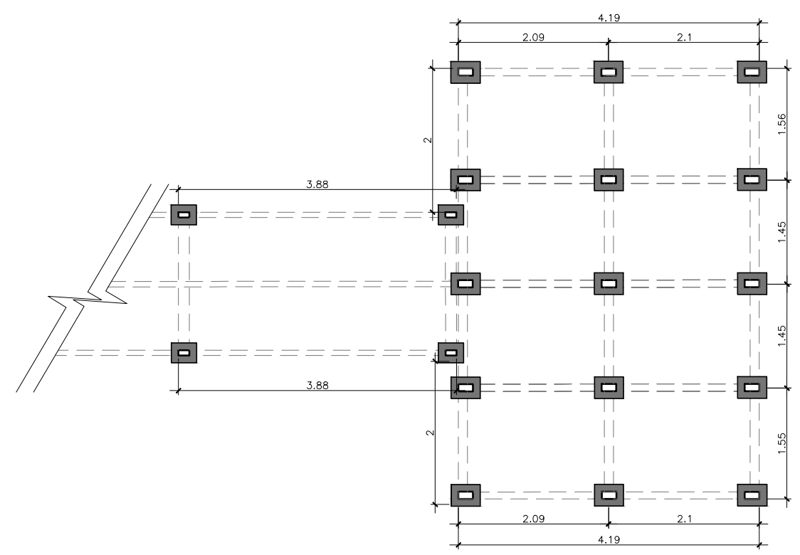
PLANTA PASARELA - MIRADOR- C 01 ESC : 1/75
