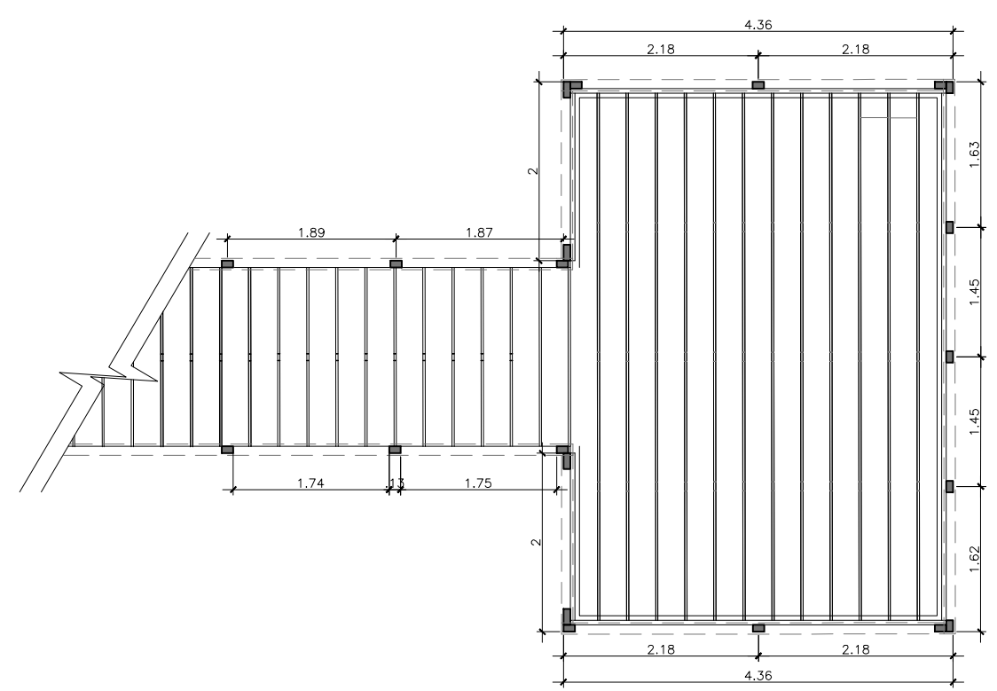
PLANTA PASARELA - MIRADOR- C 02 ESC : 1/75
