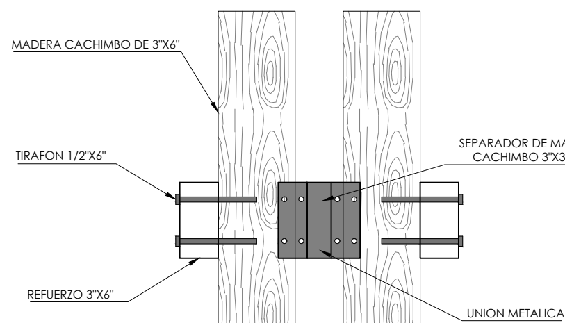
DETALLE 7 ESC:1/10
