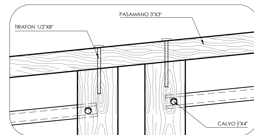
DETALLE 4 ESC:1/10
