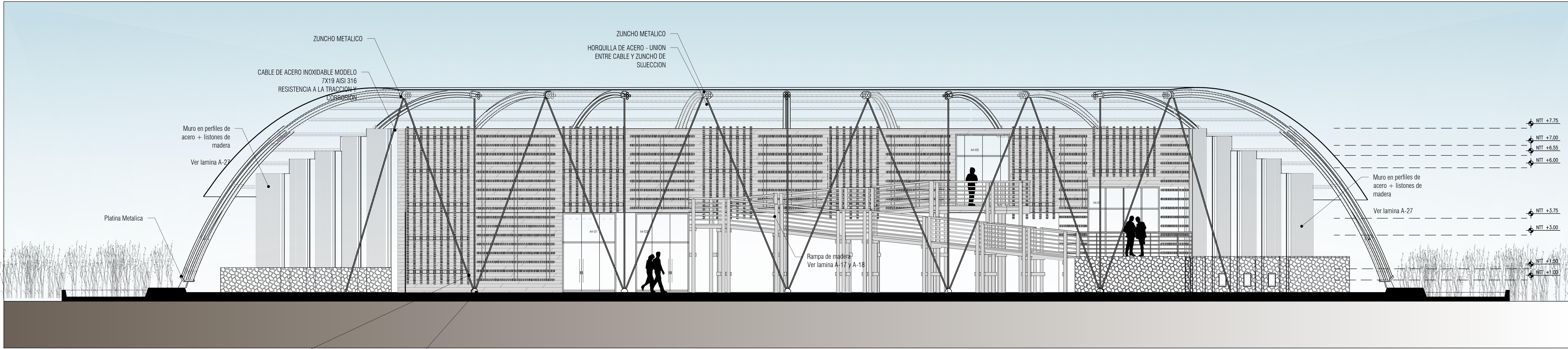
ELEVACION E-01 / SECTOR INTERPRETACION
