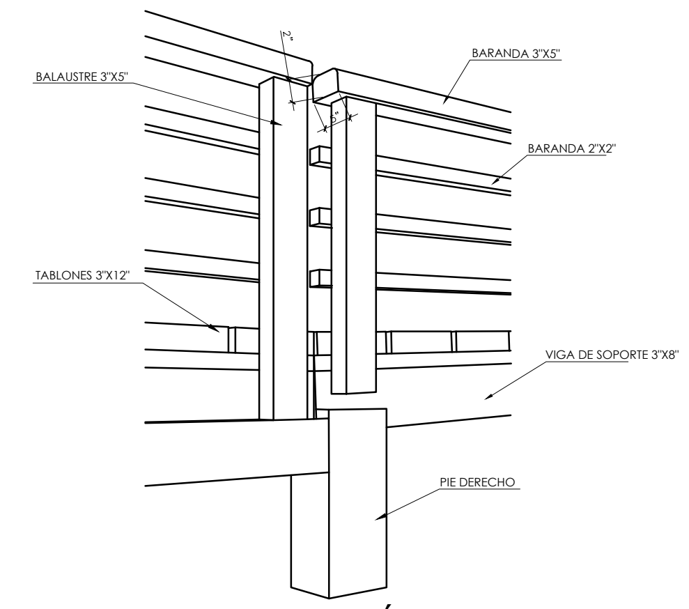
VISTA ISOMÉTRICA VISTA V-2
