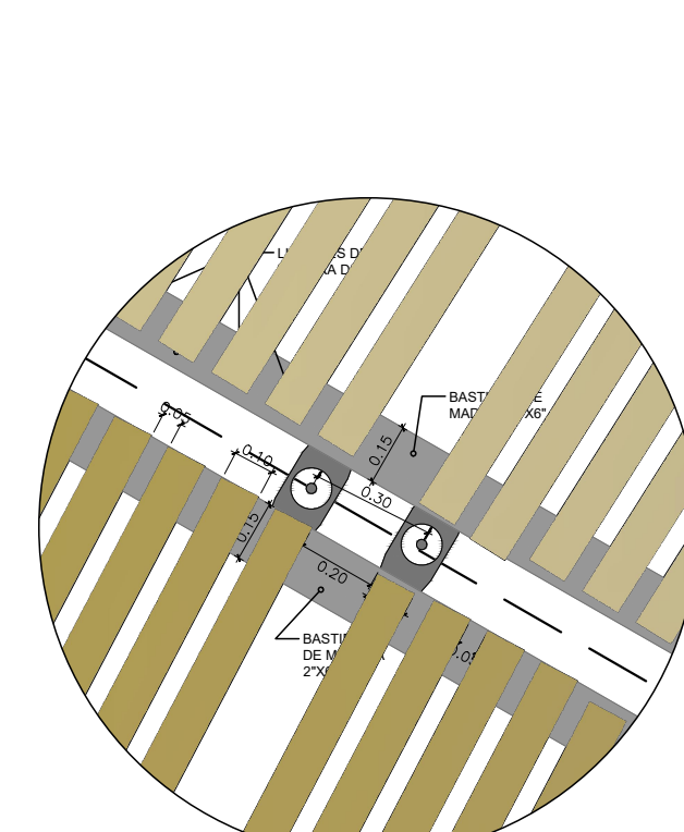
VISTA DE LISTONES DE MADERA SOBRE BASTIDORES
