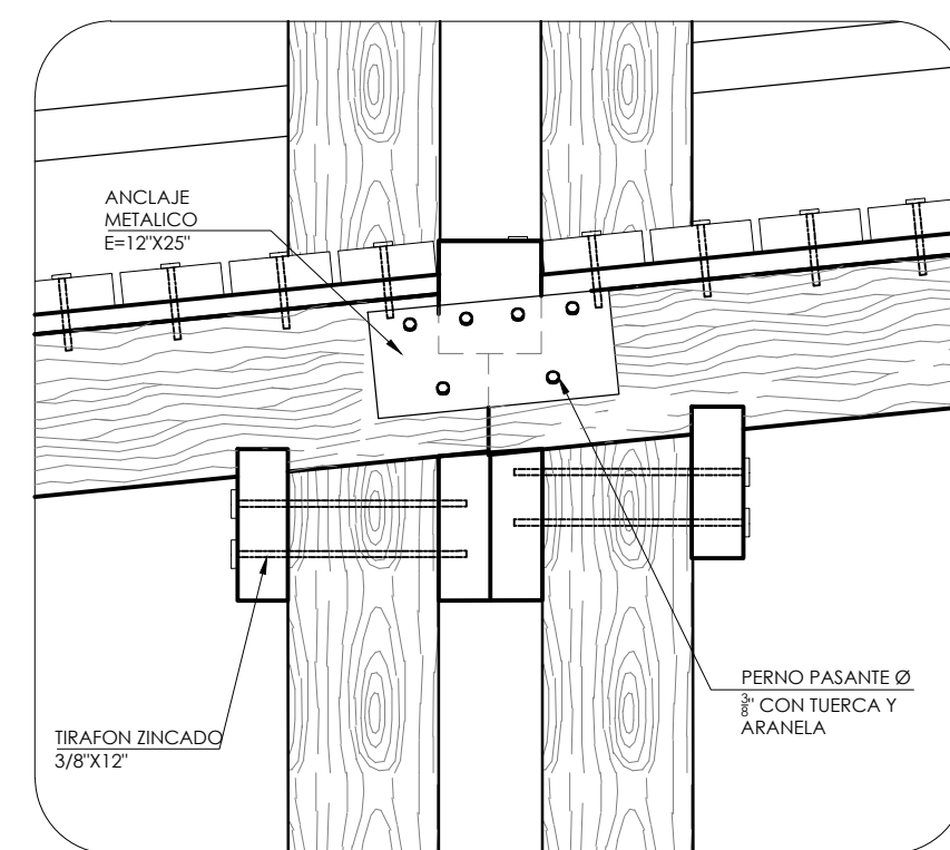
DETALLE 7 ESC:1/10
