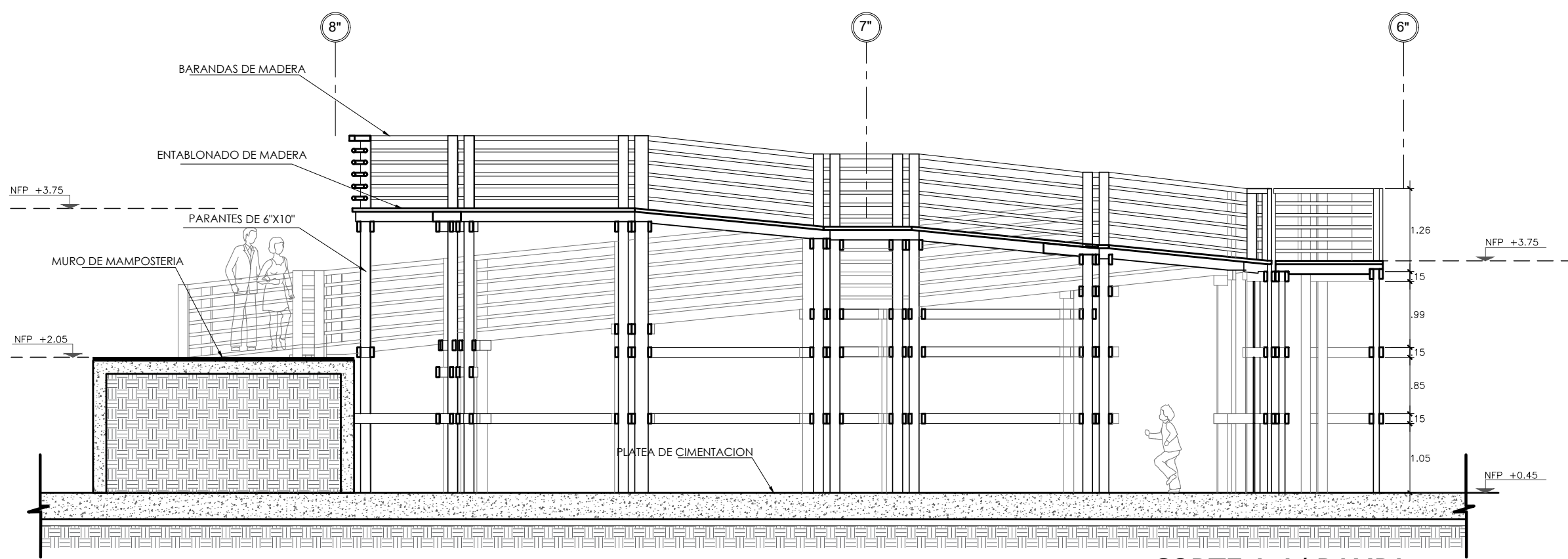
CORTE A-A/ RAMPA ESC : 1/75
