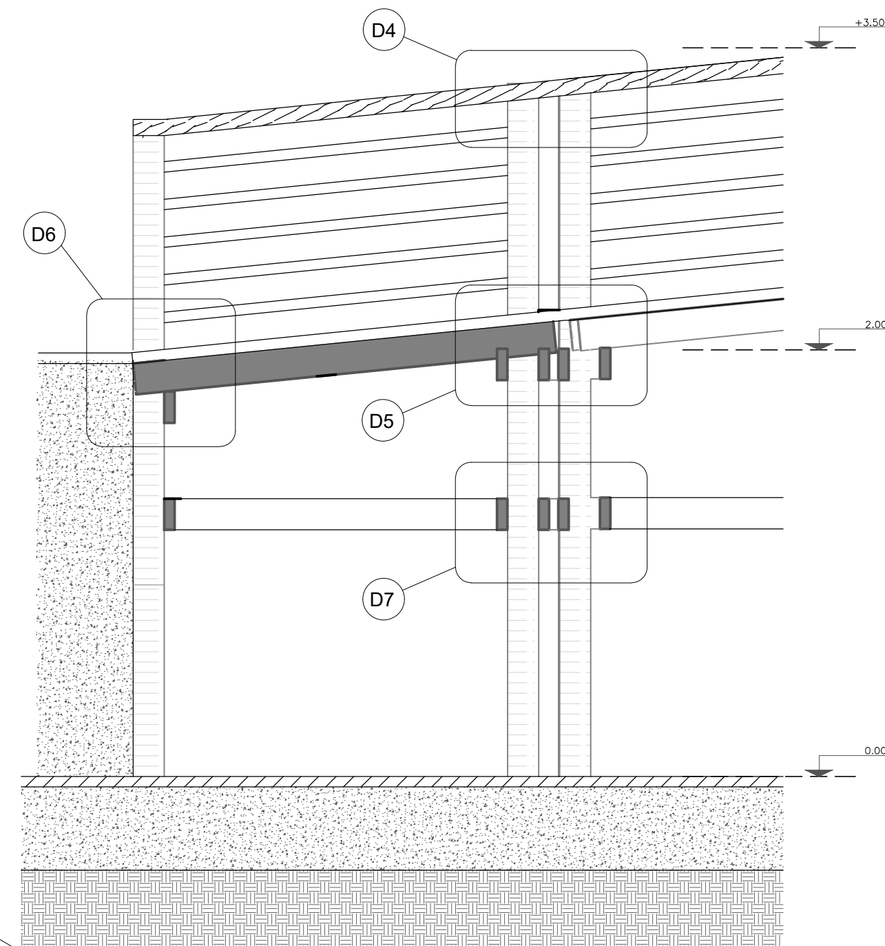
PLANTA PASARELA MIRADOR ESC : 1/25
