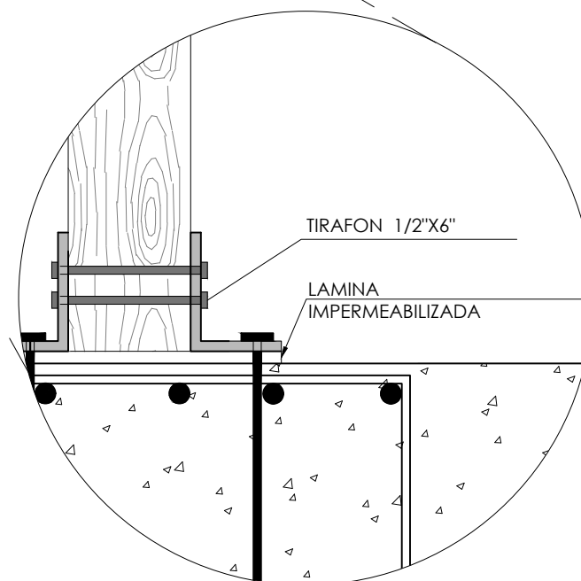
DETALLE 3 ESC:1/10
