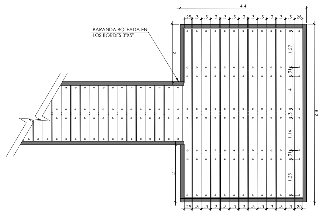
PLANTA PASARELA - MIRADOR- C 03 ESC : 1/75
