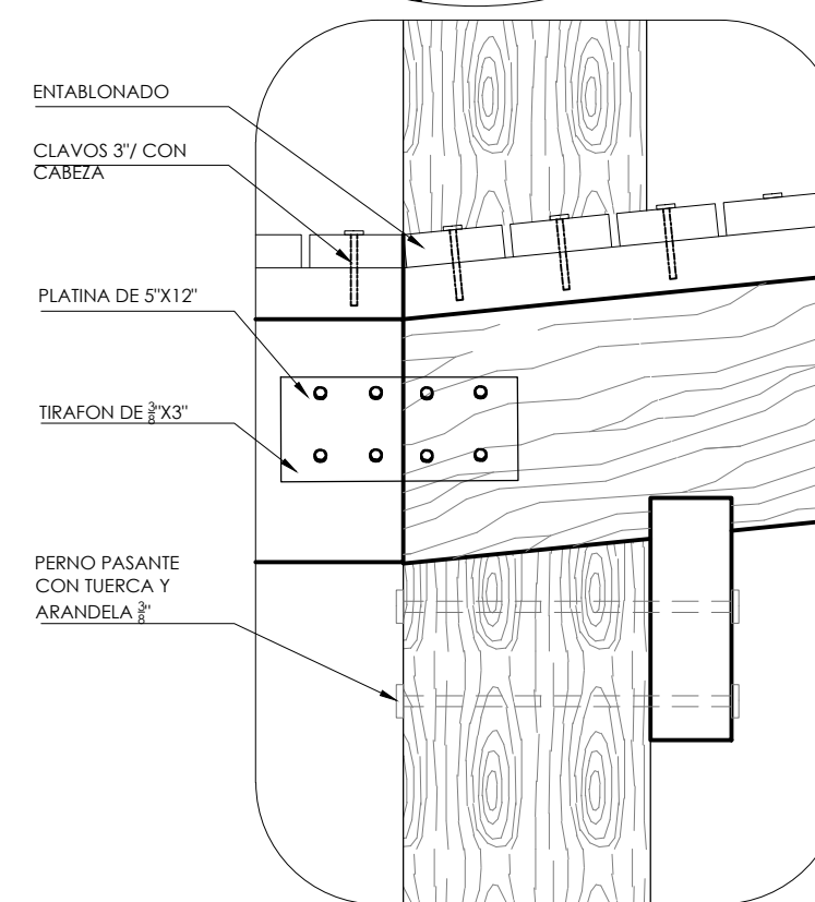
DETALLE 6 ESC:1/10
