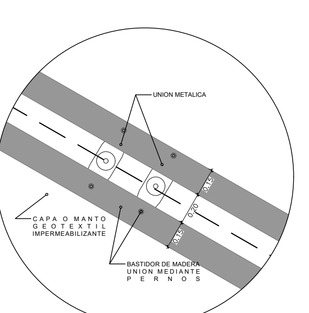
VISTA DE BASTIDORES UNIDOS MEDIANTE UNION METALICA
