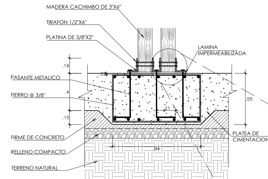
DETALLE 3 ESC:1/10
