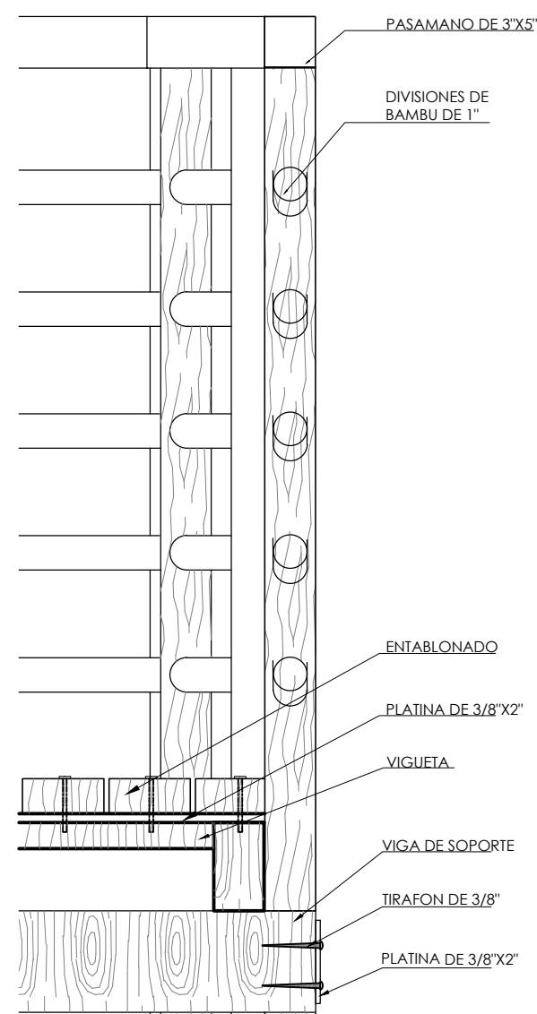
DETALLE 2 ESC:1/10
