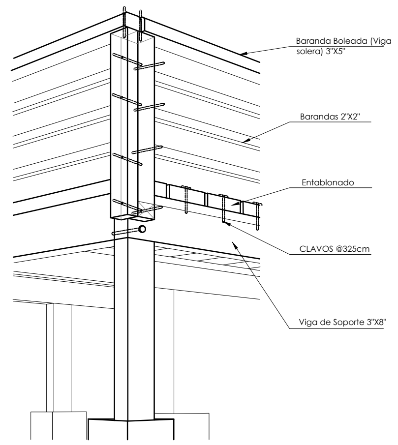
VISTA ISOMÉTRICA VISTA V-1
