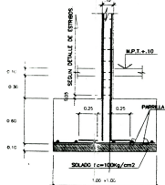
DETALLE DE ZAPATA CORTE Z-Z ESC. 1/25
