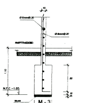
ELEVACION DE MURO CORTE 3-3
