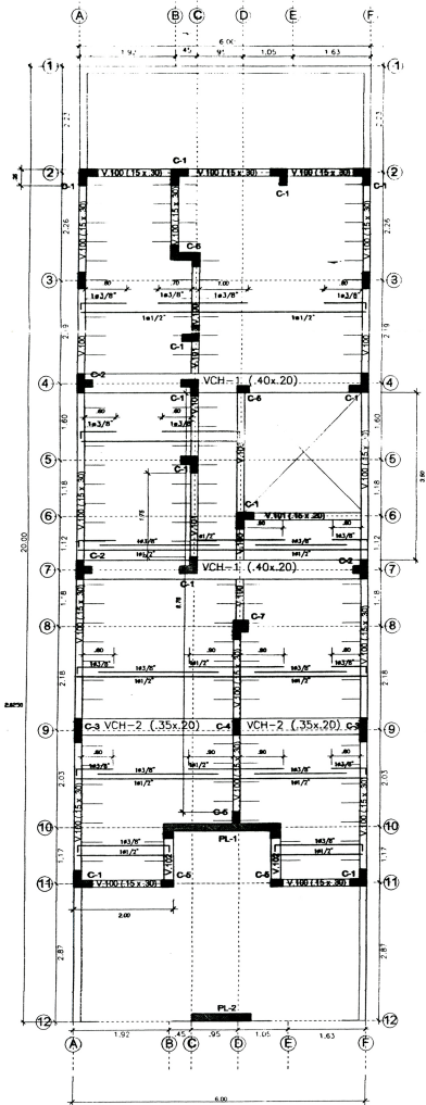
ALIGERADO 1ero al 5 to ESC: 1/75
