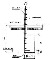
ELEVACION DE MURO CORTE 1-1
