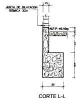
CORTE L-L
