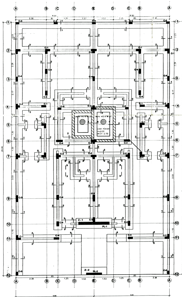
CIMENTACION ESC. 1/75
