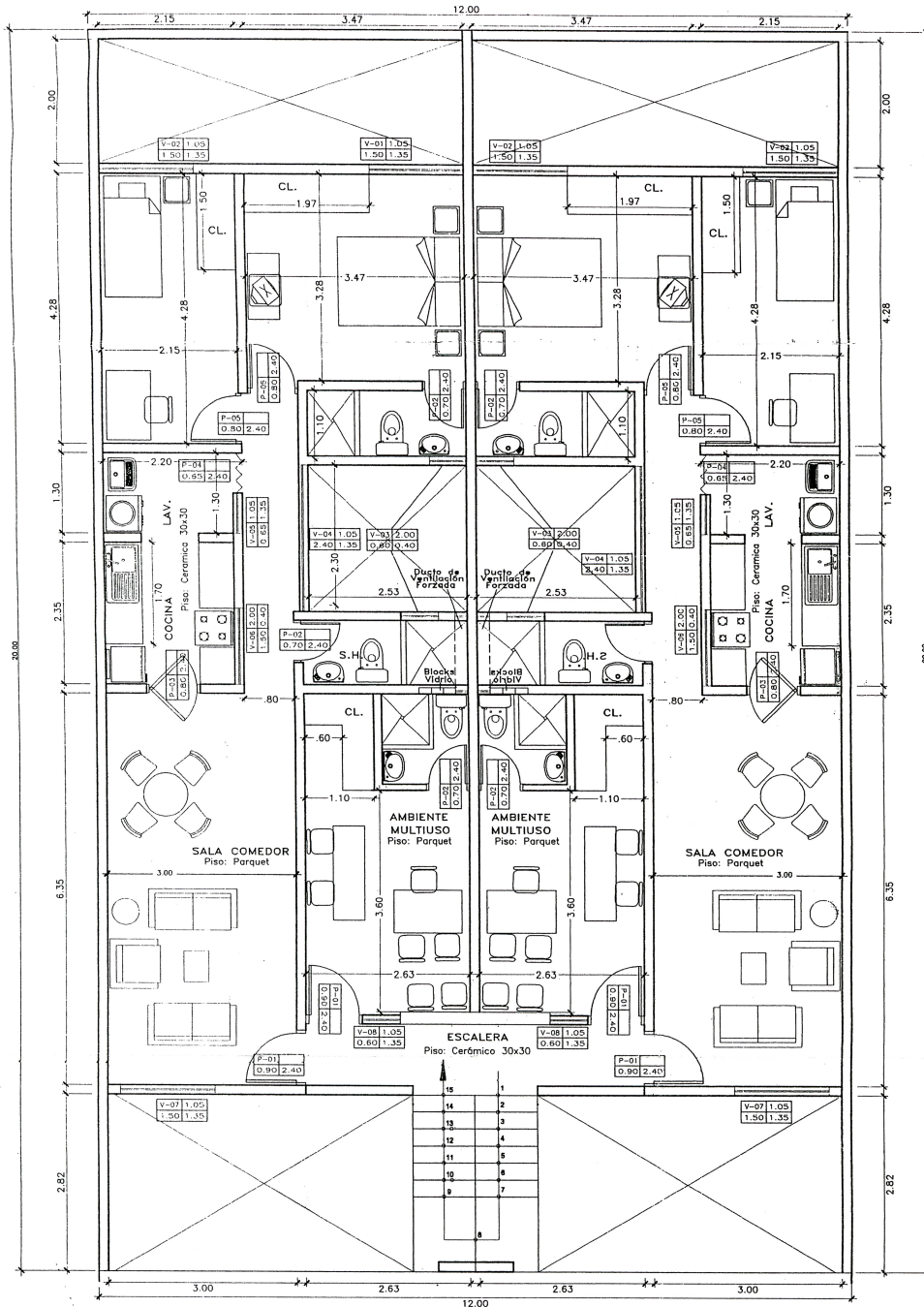
01 PLANTA 1ER PISO
