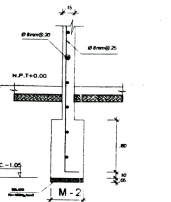
ELEVACION DE MURO CORTE 2-2
