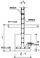
ELEVACION DE PLACA CORTE X-X ESC. 1/25
