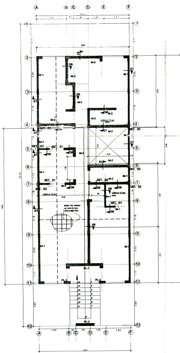
CIMENTACION (Esc. 1/75)
