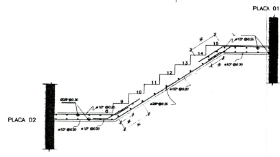
DETALLE DE ESCALERA ESC. 1/25
