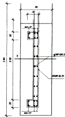
PLANTA PL-1
